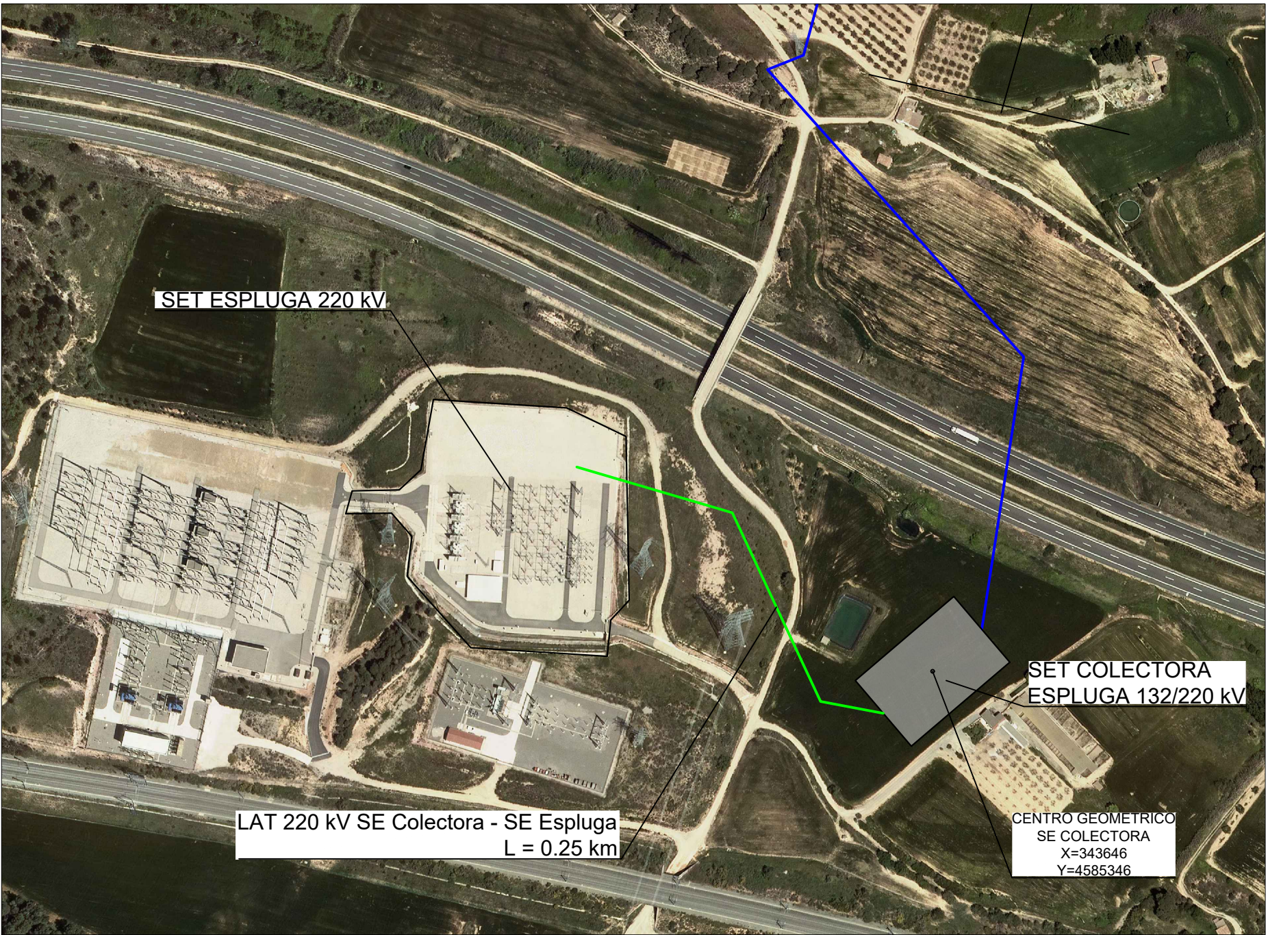
DETALLE CONEXIÓN A SUBESTACIÓN ESPLUGA 220 kV
