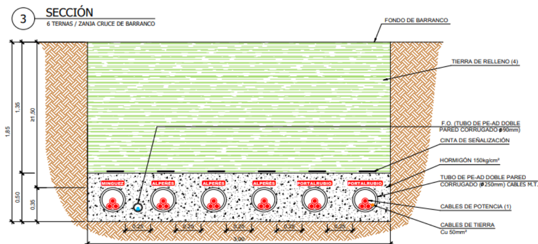
Figura 1: Sección tipo zanjas en cruce con cauces. Fuente. documentación aportada
